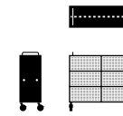
Shift+ Landscape mit 2 beidseitig bestückbaren Modulen mit je 2 Einlegeböden with 2 modules which can be configured on both sides, each with 2 shelf inserts
